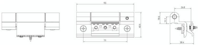
02-014-162-HOPO-00035 บานพับ Hinge HOPO Silver
