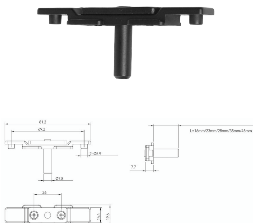
02-003-017-HOPO-00013 ตัวที C Groove HOPO Black
