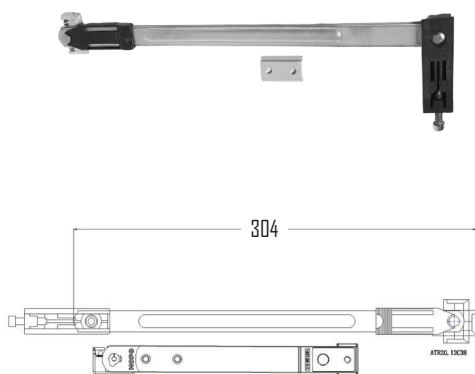
02-006-161-HOPO-00061 แขนค้ำบานปิด 12" HOPO Zinc
